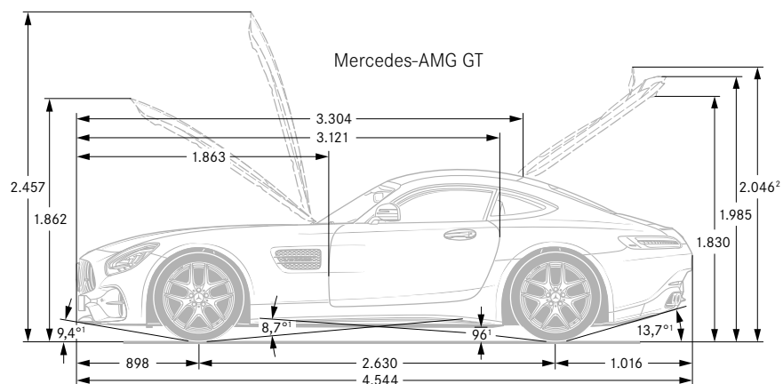
1 Bei zulässigem Gesamtgewicht 2 Spoiler ausgefahren Maße Mercedes-AMG GT S/GT C geringfügig abweichend
