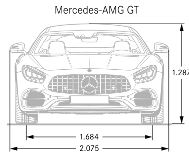
Maße Mercedes-AMG GT S/GT C geringfügig abweichend
