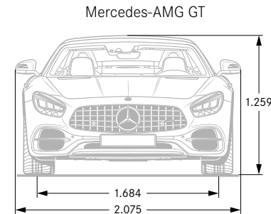
Maße Mercedes-AMG GT S geringfügig abweichend
